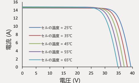
I-V 曲線 (455 W)
