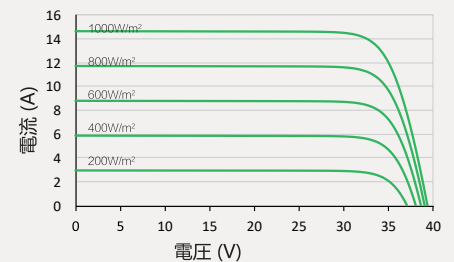
P-V 曲線 (455 W)
